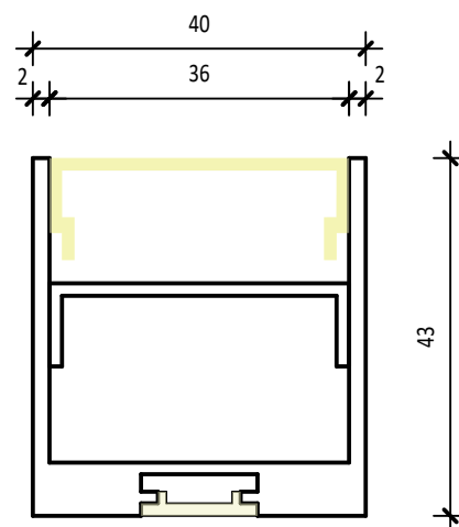
Diffusor BÜNDIG
